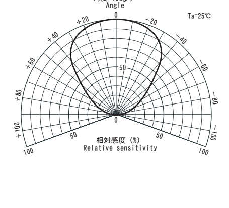
■指向特性
